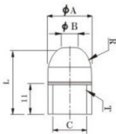
半圓型 Domed type
