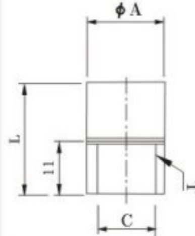
平型 Flat type
